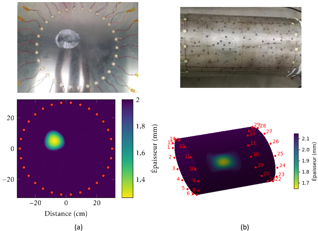
Figure 1 : Tomographie par ondes élastiques guidées expérimentale (a) dans une plaque, (b) dans un tube.
